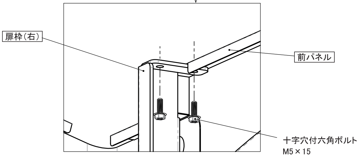
【庫内側から見た図】
