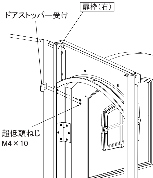
【庫内側から見た図】
