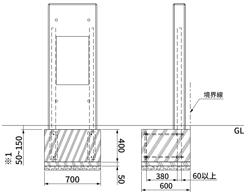
偏心基礎金具セットB 2セット分
