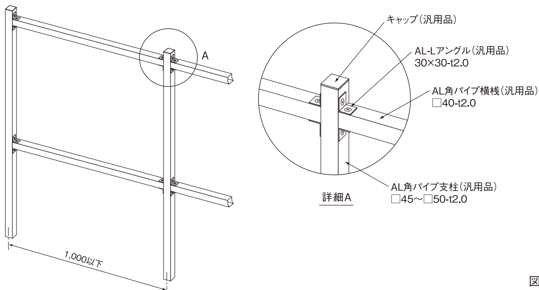
支柱・横棧組立図(参考例)
